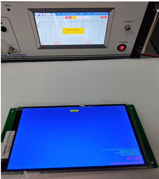
图 5-4 群脉冲测试图
