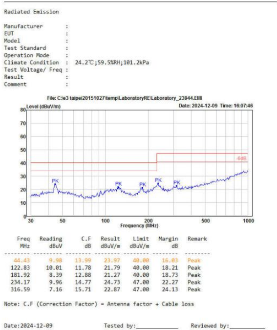
图 5-6 辐射测试水平方向
